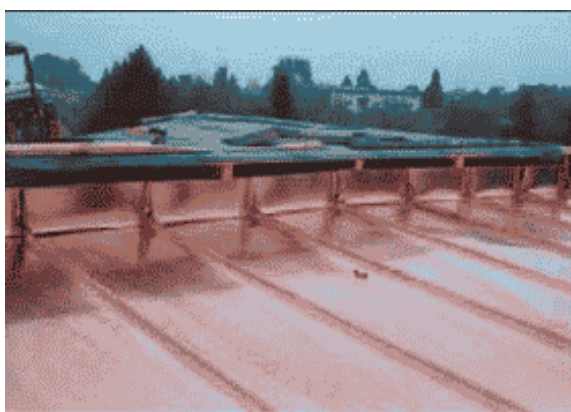
Рис. 7. Фальцевая кровля
